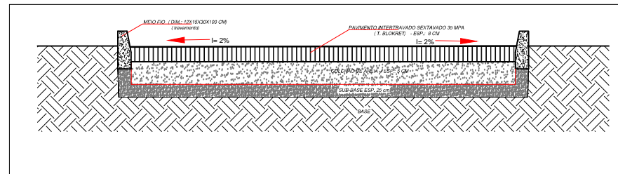
CORTE AA' ESC: S/E
