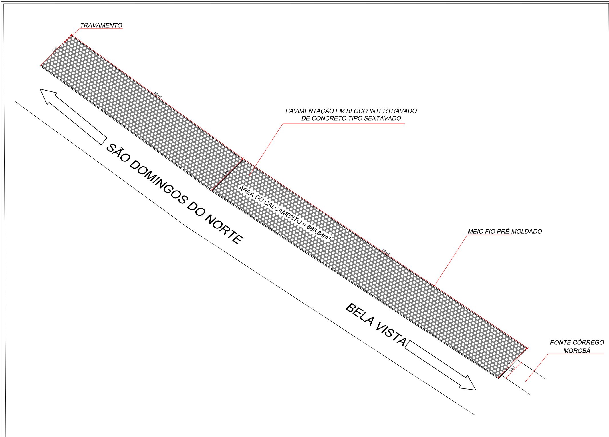
PLANTA BAIXA - PAVIMENTAÇÃO ESC: 1/200
